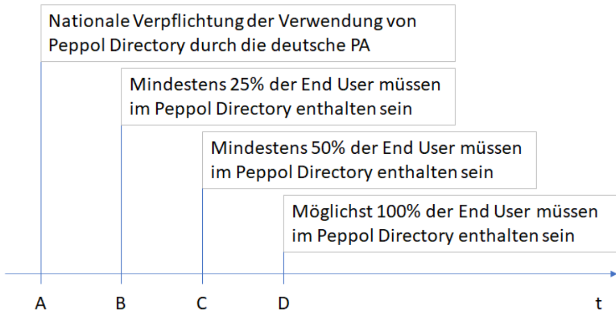
Abbildung 1: Migrations-Modell
